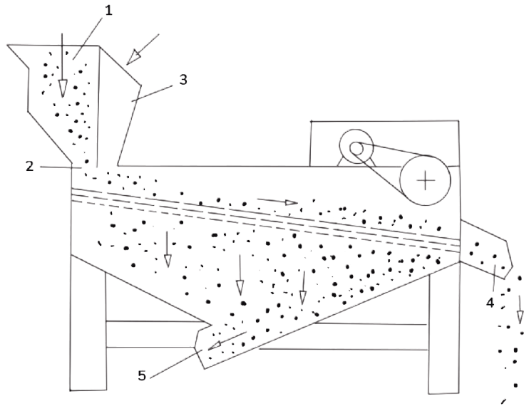
Gambar 6.23 Sketsa mesin sortasi biji-bijian. Sumber: fao.org
