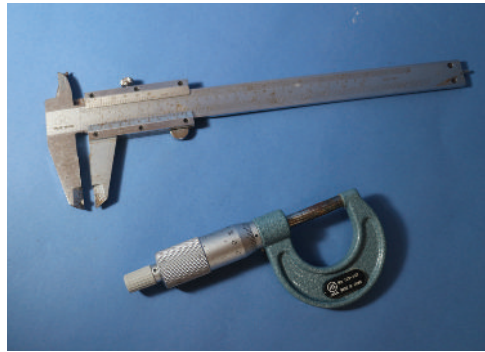
Gambar 4.28 Jangka sorong dan mikrometer. Sumber: Wagiyono/2022
