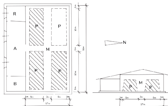
Gambar 6.24 Sketsa tata letak bangunan gudang. Sumber: fao.org
