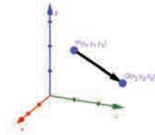
Gambar 3.20 Vektor PQ
